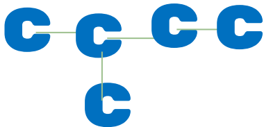
2,metil butana
