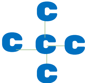
2,2 metil propana
